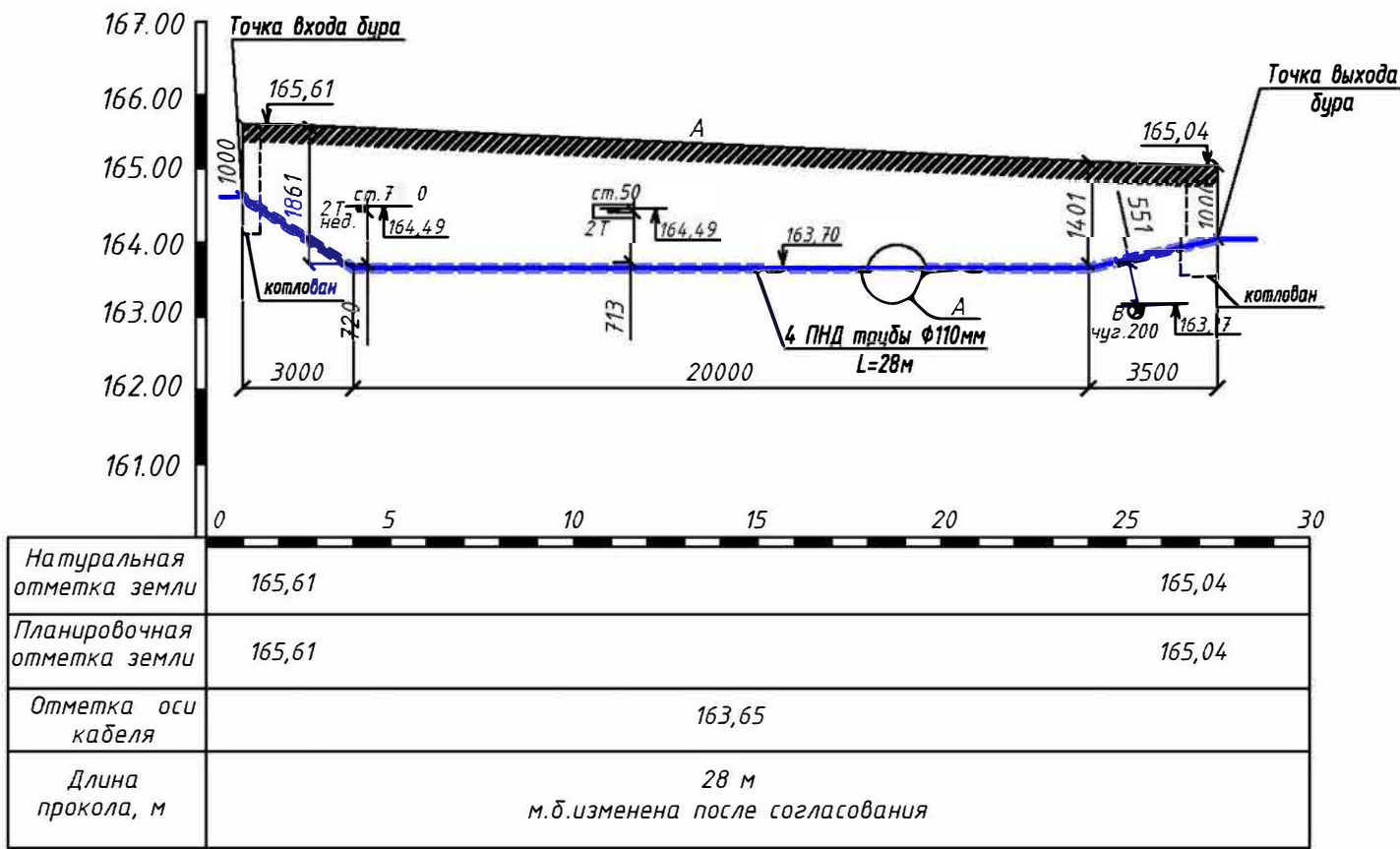
ПРОКОЛ №1 по вертикали М 1:100 по горизонтали М 1:200
